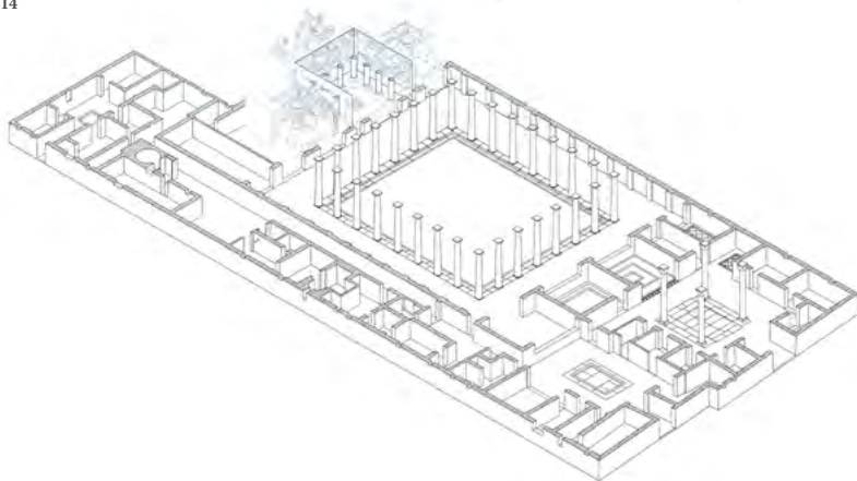
14 Spaccato assonometrico della Casa del Labirinto a Pompei (Mazzoleni, 2004)
